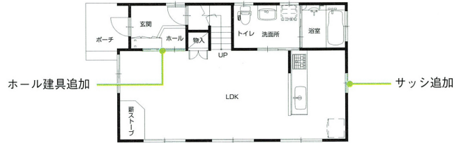
1F 平面図
