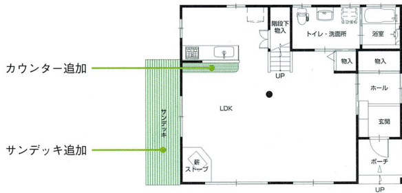
1F 平面図
